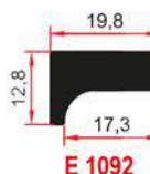
E 1092 0,420 Kg/m
