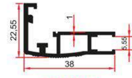
SM 1006 A 0,405 Kg/m
