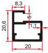
E 6029 0,265 Kg/m
