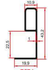
7574 0,265 Kg/m
