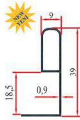
1010 P EKO 0,215 Kg/m
