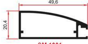
SM 1001 0,475 Kg/m
