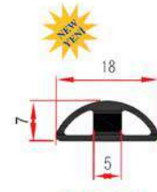
PRF-30326 0,180 Kg/m
