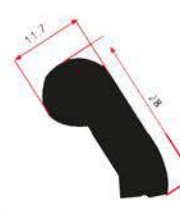
SM 6013 A 0,615 Kg/m
