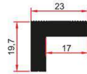
SM 6013 M 0,595 Kg/m
