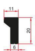
E 1382 0,395 Kg/m
