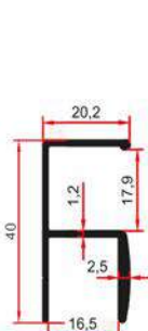
SM 1013 BF 0,365 Kg/m
