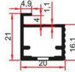
SM 1007 E 0,275 Kg/m
