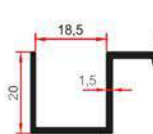
9435 0,335 Kg/m
