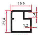
10954 0,275 Kg/m
