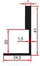
9126 A 0,445 Kg/m
