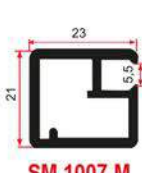
SM 1007 M 0,400 Kg/m
