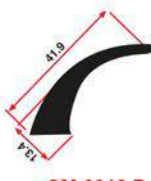
SM 6013 B 0,665 Kg/m
