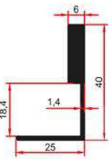
7503 0,485 Kg/m
