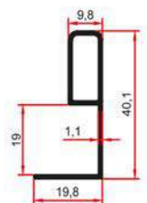
8780 0,275 Kg/m
