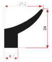
E 1656 0,520 Kg/m
