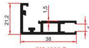
SM 1006 B 0,445 Kg/m
