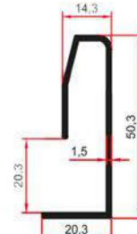
SM 1013 Y 0,425 Kg/m
