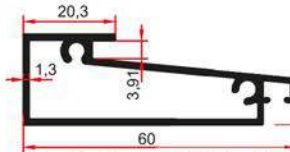
Pvc Doğrama Eşik Profili 8032 0,615 Kg/m
