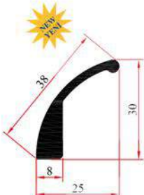
PRF-30165 0,465 Kg/m
