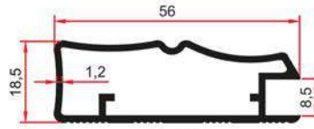
SM 1000 C 0,545 Kg/m
