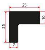
SM 6014 BK 1,005 Kg/m
