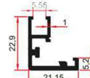
SM 1005 A 0,275 Kg/m
