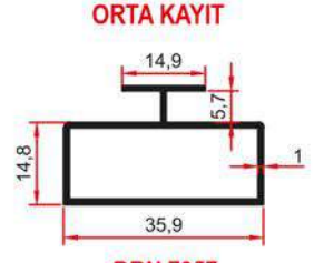
BRN 7357 0,315 Kg/m
