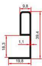
SM 1010 P 0,275 Kg/m
