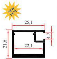
PRF-30407 0,490 Kg/m
