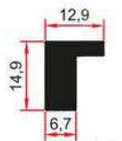
E 1014 0,320 Kg/m
