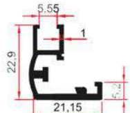
SM 1005 0,285 Kg/m
