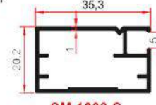
SM 1003 C 0,375 Kg/m
