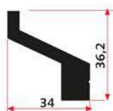
SM 6013 J 0,980 Kg/m
