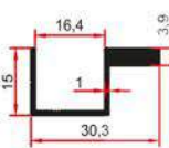
8965 0,255 Kg/m
