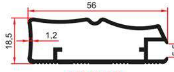
SM 1000 B 0,545 Kg/m
