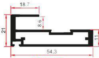
SM 1002 E 0,720 Kg/m
