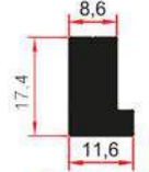
SM 6014 CR 0,445 Kg/m
