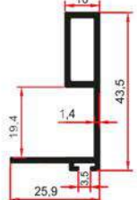
6622 0,405 Kg/m
