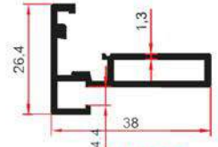
SM 1005 B 0,435 Kg/m
