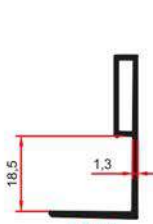
8800 0,305 Kg/m
