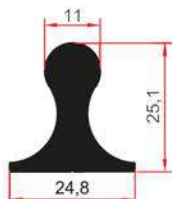
SM 6013 G 0,695 Kg/m
