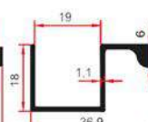
8781 0,295 Kg/m
