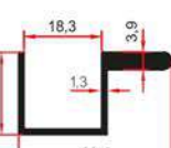
7405 0,345 Kg/m
