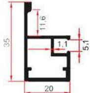
7356 0,365 Kg/m
