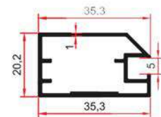
SM 1003 A 0,365 Kg/m
