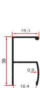
3796 A 0,235 Kg/m
