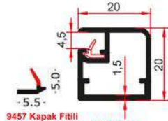
2189 A 0,315 Kg/m
