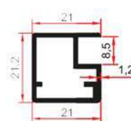
SM 1007 N 0,305 Kg/m
