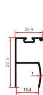
9476 0,295 Kg/m
