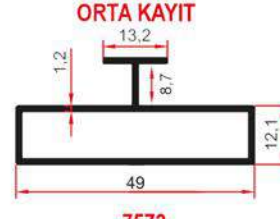
7573 0,450 Kg/m
