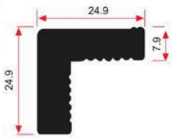
E 1391 0,880 Kg/m
