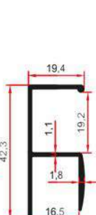
6066 0,305 Kg/m
