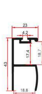
1013 BJ 0,435 Kg/m
