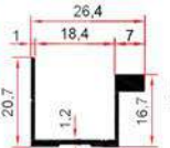
1936 0,240 Kg/m
