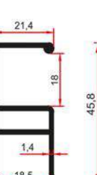
SM 1013 0,485 Kg/m
