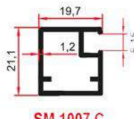
SM 1007 C 0,295 Kg/m
