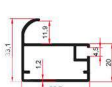
11383 A 0,455 Kg/m
