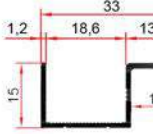
9382 0,230 Kg/m
