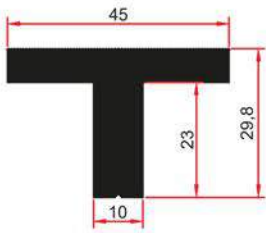
SM 6013 I 1,425 Kg/m
