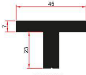
SM 6013 H 1,470 Kg/m
