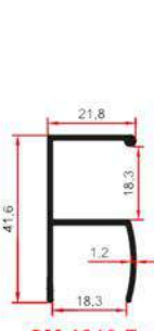
SM 1013 F 0,335 Kg/m
