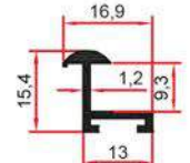
2847 0,135 Kg/m
