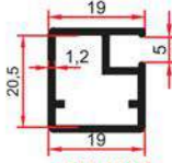
SM 1007 0,275 Kg/m
