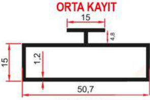
SM 1007 B 0,465 Kg/m
