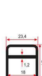
SM 1012 0,410 Kg/m
