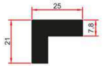
E 1068 0,805 Kg/m
