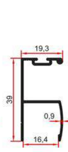
3797 A 0,255 Kg/m
