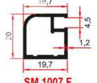
SM 1007 F 0,265 Kg/m
