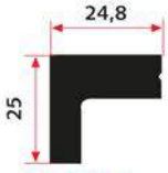
SM 6013 İ 0,950 Kg/m
