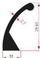
E 1077 0,435 Kg/m
