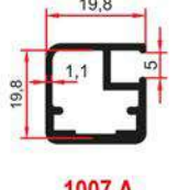
1007 A 0,315 Kg/m
