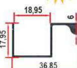
7505 EKO 0,290 Kg/m
