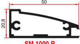
SM 1000 B 0,570 Kg/m
