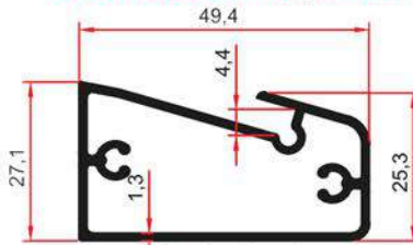
Bombe Kapak 5547 0,655 Kg/m
