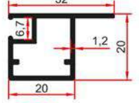
9741 0,315 Kg/m
