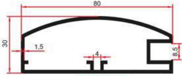
SM 1001 C 0,955 Kg/m
