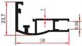
SM 1006 0,415 Kg/m
