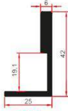
8755 0,615 Kg/m
