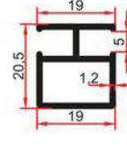
SM 1007 T 0,285 Kg/m
