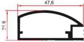
SM 1001 D 0,535 Kg/m
