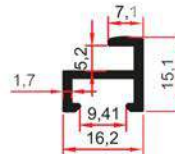
SM 1002 ÇR 0,185 Kg/m LÜKS RESİM ÇERÇEVESİ
